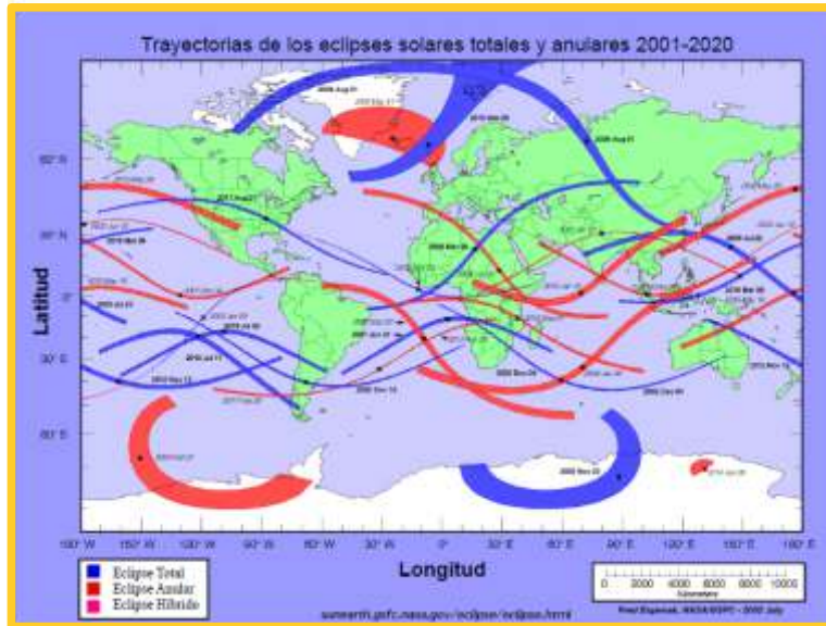
Fig. 17. Trayectorias de los eclipses solares totales y anulares desde 2001 a 2020.
