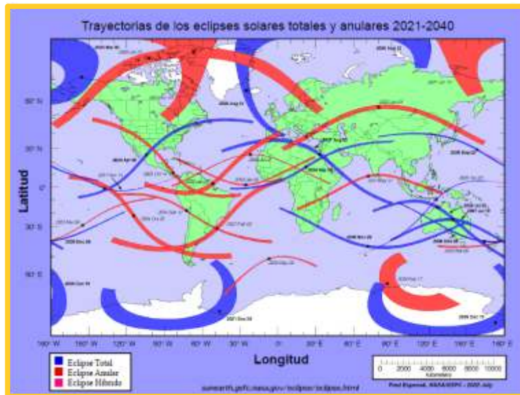
Fig. 18. Trayectorias de los eclipses solares totales y anulares desde 2021 a 2040.
