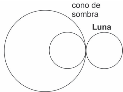
Fig. 20b. Midiendo el diámetro de la Luna.
